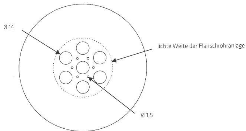
Bild 1: Mustervorlage für elektrisch nichtleitende Flachdichtungsmaterialien
